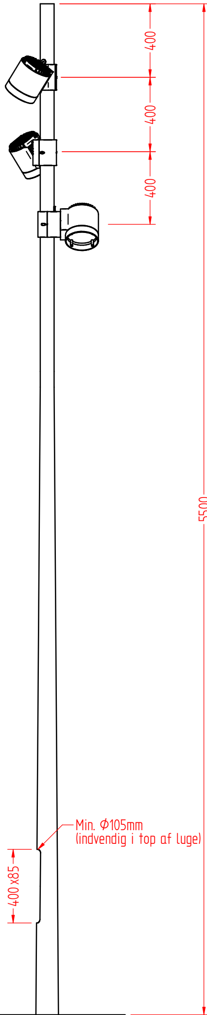
5,5 m mast: 3,5 m konisk + 2 m forlængerrør, \phi 76 mm - for 3 armatur
