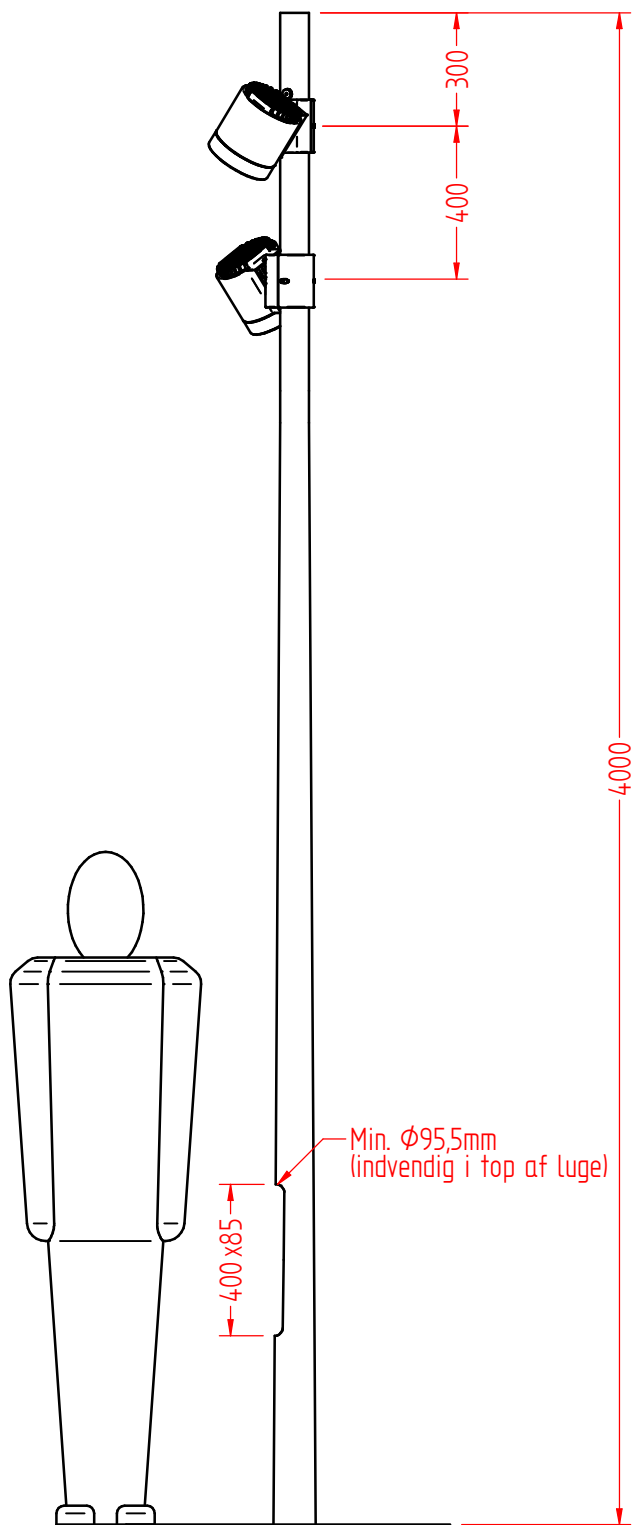
4 m mast: 3 m konisk + 1 m forlængerrør, \phi 76 mm - for 2 armatur
