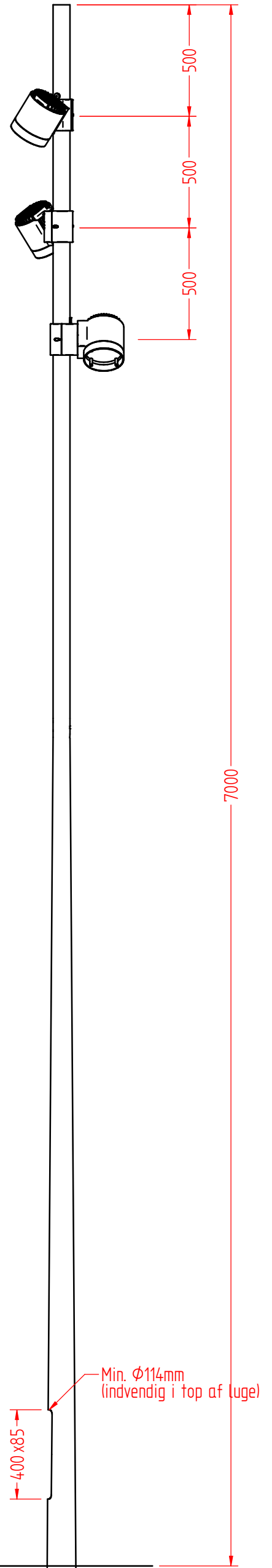
7 m mast: 4 m konisk + 3,2m forlængerrør, \phi 76 mm - for 3 armatur (7m maste nedgraves 1m)
